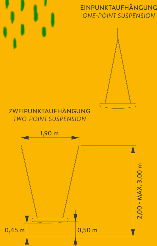
AUFHÄNGEVARIANTEN NESTSCHAUKELN SUSPENSION OPTIONS FOR NEST SWINGS
